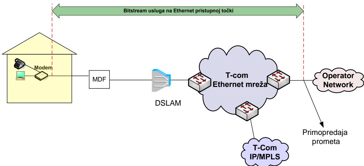
Slika 14. Veleprodajni širokopolasni pristup za pružanje VoIP usluge na Ethernet razini u slučaju kada krajnji korisnik ostvaruje Osnovni pristup mreži putem usluge Operatora korisnika
