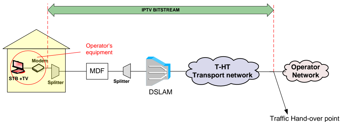
Slika 19. Koncept posebnog virtualnog kanala za IPTV uslugu u slučaju kada Krajnji korisnik ostvaruje Osnovni pristup mreži putem usluge T-Coma
