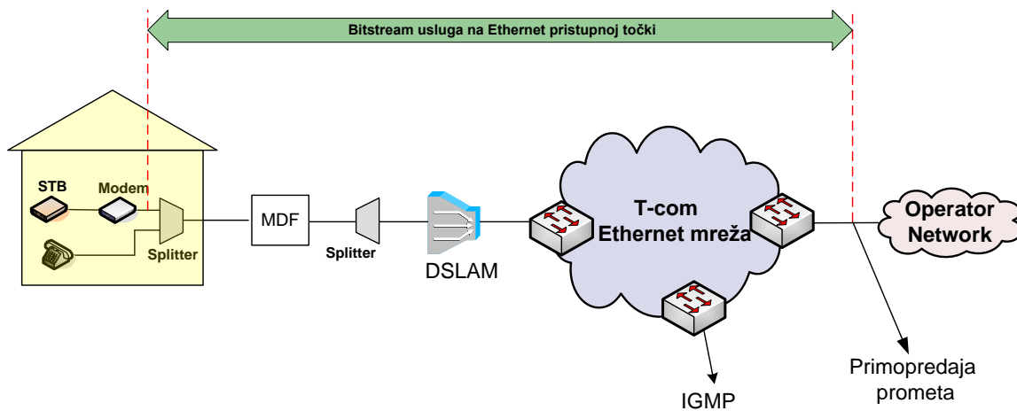
Slika 23. IPTV usluga na Ethernet razini putem ADSL/VDSL tehnologije u slučaju kada Krajnji korisnik ostvaruje Osnovni pristup mreži putem usluge T-Coma
