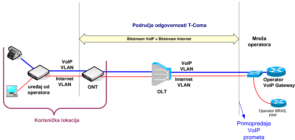
Slika 17. Veleprodajni širokopojasni pristup za pružanje VoIP usluge preko FTTH pristupa (GPON) na OLT razini
