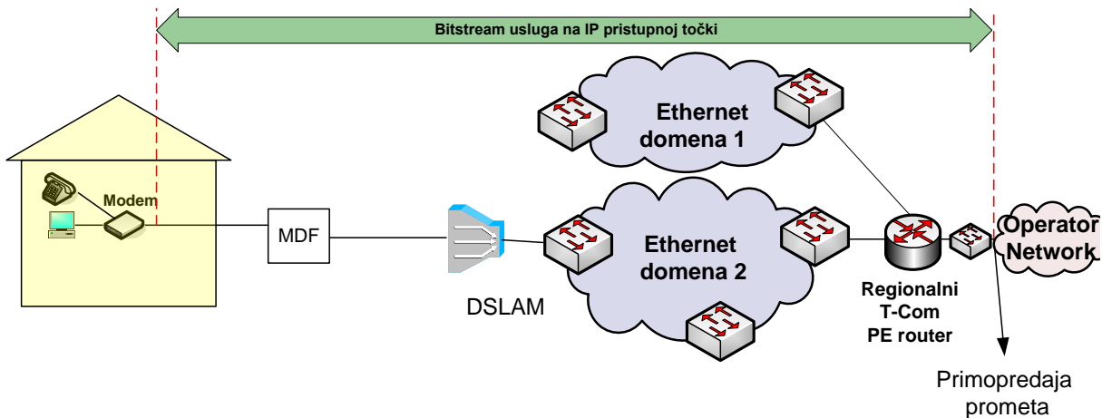
Slika 15. Veleprodajni širokopoljasni pristup za pružanje VoIP usluge na IP razini u slučaju kada Krajnji korisnik ostvaruje Osnovni pristup mreži putem usluge T-Coma
