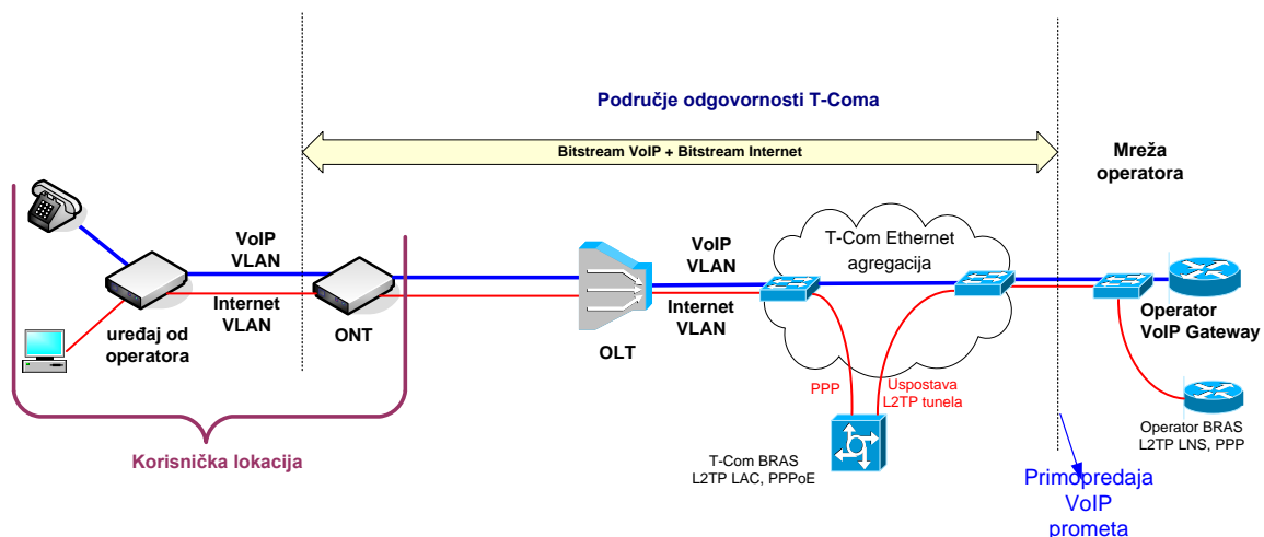
Slika 12. Realizacija posebnog virtualnog kanala za VoIP uslugu preko FTTH pristupa (GPON)
