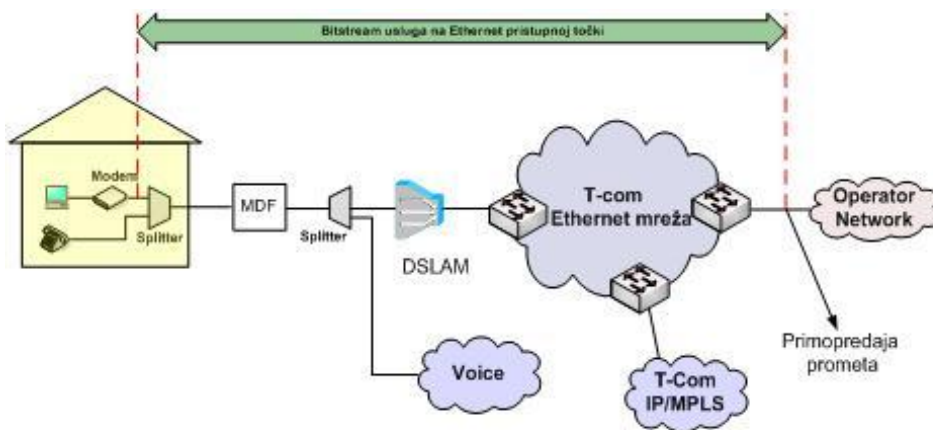
Slika 3. Veleprodajni širokopojasni pristup za pružanje Internet usluge na Ethernet razini u slučaju kada Krajnji korisnik ostvaruje Osnovni pristup mreži putem usluge T-Coma.
