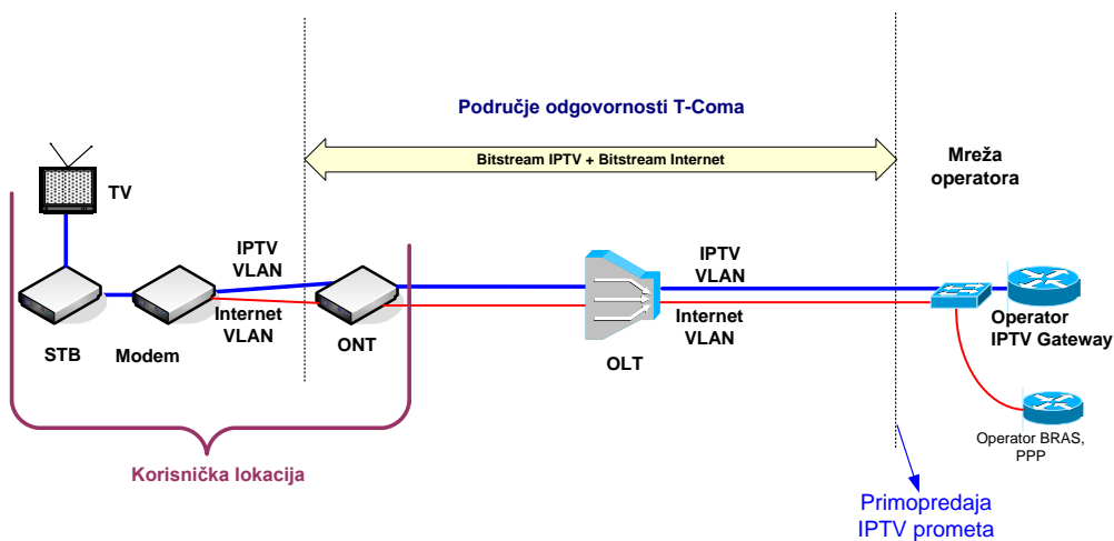
Slika 25. Veleprodajni širokopojasni pristup za pružanje IPTV usluge preko FTTH pristupa (GPON) na OLT razini
