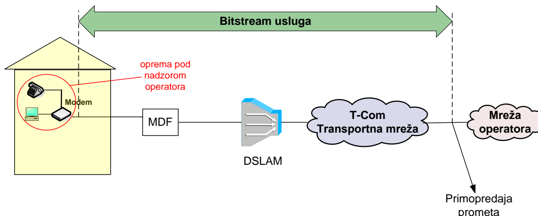
Slika 10. Koncept posebnog virtualnog kanala za VoIP uslugu u slučaju kada Krajnji korisnik ostvaruje Osnovni pristup mreži putem usluge Operatora korisnika
