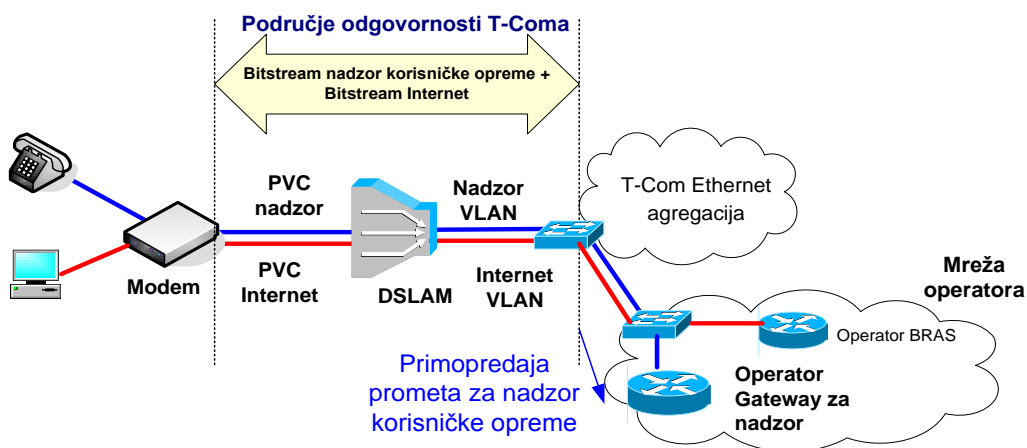
Slika 28. Veleprodajni širokopojasni pristup za pružanje usluge nadzora korisničke opreme preko ADSL/VDSL pristupa na DSLAM razini
