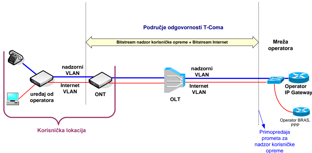
Slika 27. Veleprodajni širokopojasni pristup za pružanje usluge nadzora korisničke opreme preko FTTH pristupa (GPON) na OLT razini
