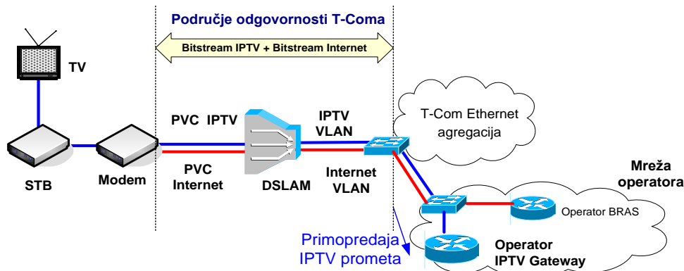
Slika 26. Veleprodajni širokopolasni pristup za pružanje IPTV usluge preko ADSL/VDSL pristupa na DSLAM razini
