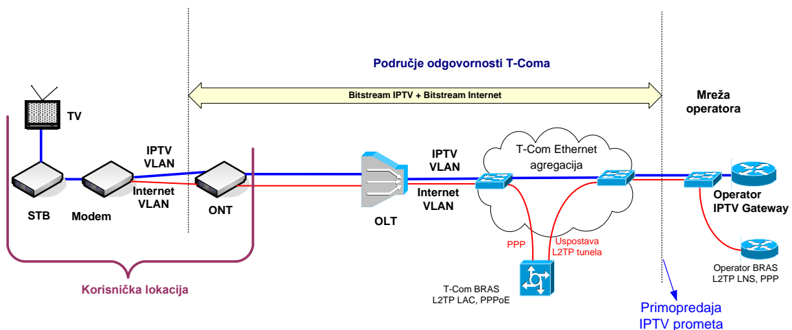
Slika 22. Realizacija posebnog virtualnog kanala za IPTV uslugu preko FTTH pristupa (GPON)
