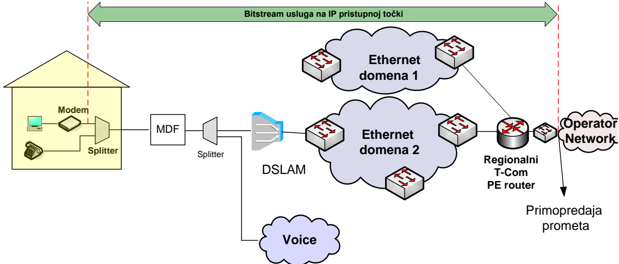
Slika 15. Veleprodajni širokopoljasni pristup za pružanje VoIP usluge na IP razini u slučaju kada Krajnji korisnik ostvaruje Osnovni pristup mreži putem usluge T-Coma
