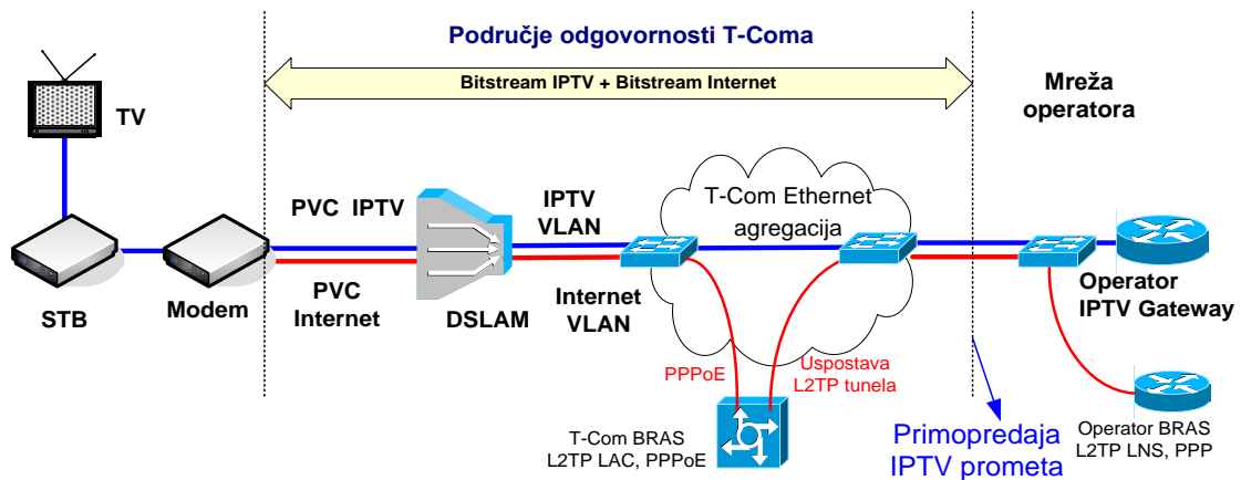
Slika 21. Realizacija posebnog virtualnog kanala za IPTV uslugu preko ADSL/VDSL pristupa (kod VDSL pristupa između modema i DSLAM-a koristi se odgovarajući VLAN)
