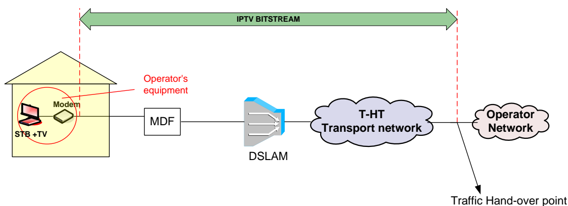
Slika 20. Koncept posebnog virtualnog kanala za IPTV uslugu u slučaju kada Krajnji korisnik ostvaruje Osnovni pristup mreži putem usluge Operatora korisnika
