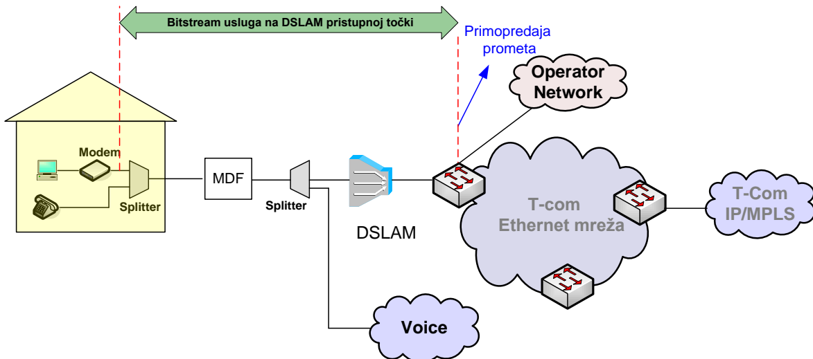
Slika 6. Veleprodajni širokopojasni pristup za pružanje Internet usluge na DSLAM razini u slučaju kada Krajnji korisnik ostvaruje Osnovni pristup mreži putem usluge T-Coma
