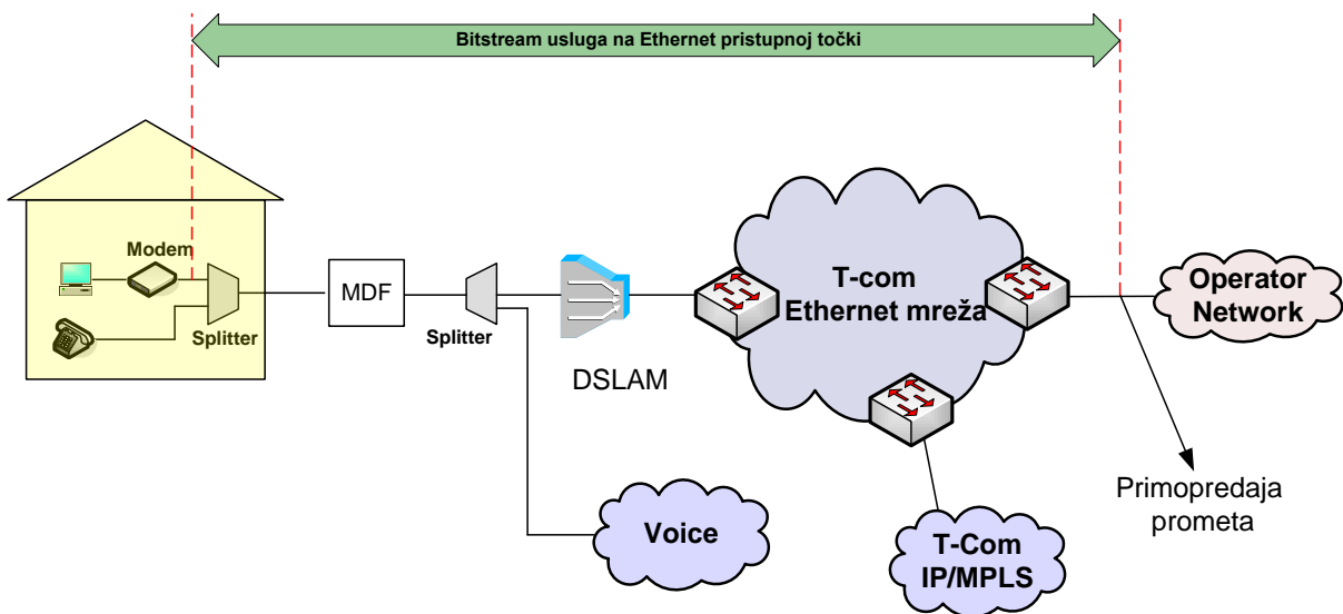
Slika 13. Veleprodajni širokopolasni pristup za pružanje VoIP usluge na Ethernet razini u slučaju kada krajnji korisnik ostvaruje Osnovni pristup mreži putem usluge T-Coma
