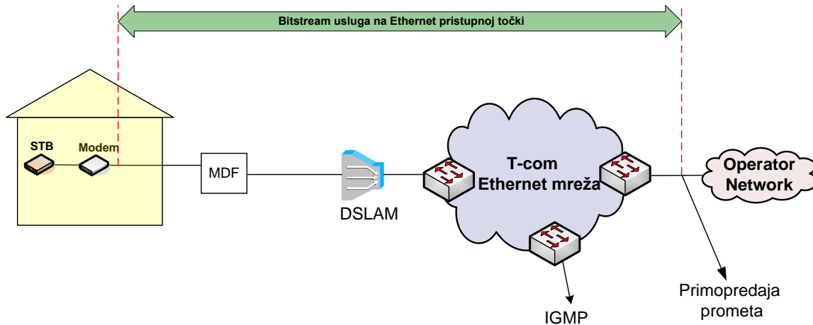
Slika 24. IPTV usluga na Ethernet razini putem ADSL/VDSL tehnologije u slučaju kada Krajnji korisnik ostvaruje Osnovni pristup mreži putem usluge Operatora korisnika
