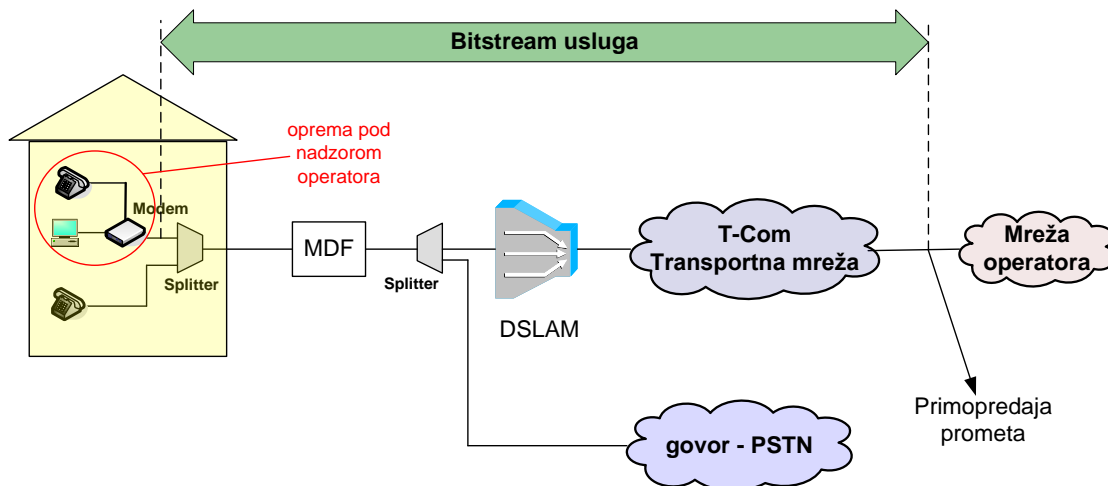
Slika 9. Koncept posebnog virtualnog kanala za VoIP uslugu u slučaju kada Krajnji korisnik ostvaruje Osnovni pristup mreži putem usluge T-Coma
